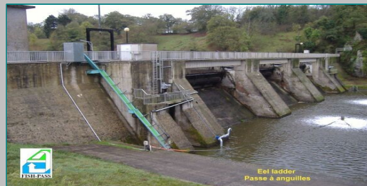
Barrage d'Apremont, Vie \Delta h = 11.50 m
